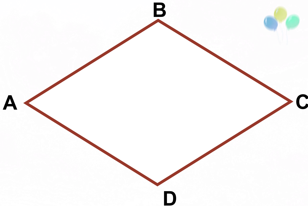
Hình thoi ABCD
