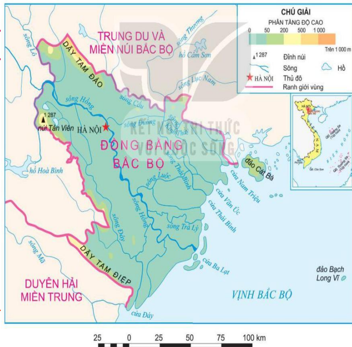
▲ Hình 2. Lược đồ địa hình vùng Đồng bằng Bắc Bộ
